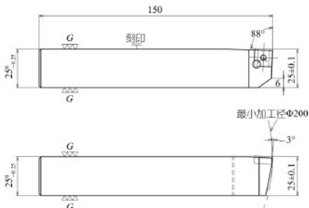
图8 自制刀具图纸
