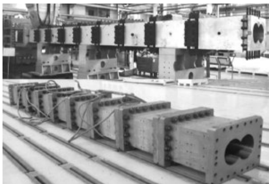
图1 同向造粒机组机筒串联组装图
