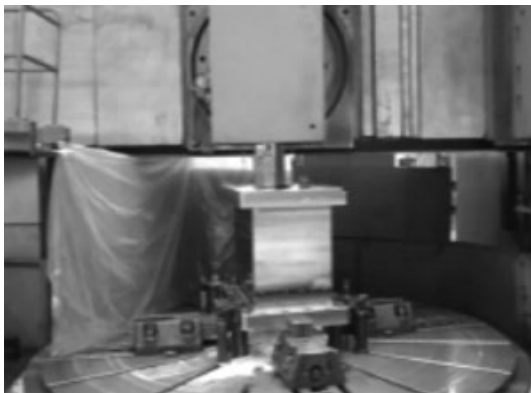
图3 数控立车磨削机筒内孔
