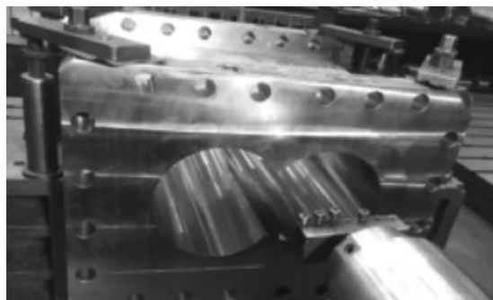
图4 数控镗床加工
